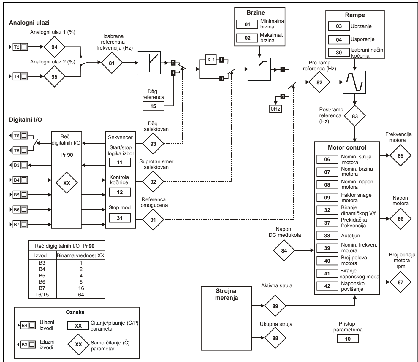
Slika 8-1 Logički diagram dijagnostike
