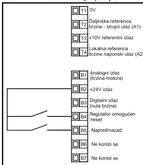
Slika 7-2 Minimalno ožičenje upravljačkih izvoda
